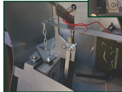
MinkPolice MP10 über Kabel mit Stelleinheit verbunden
