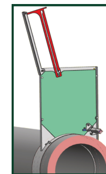
Schieber geöffnet zum Stellen der Falle
