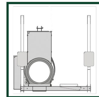
Laufrost abgesenkt
