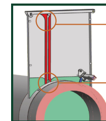
Schieber geschlossen, Waschbärsicherung aktiv
