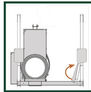
Laufrost hochgeklappt
