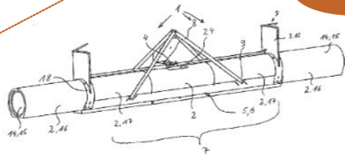
Entwicklung der ersten Vollmobilen Betonrohrfalle
