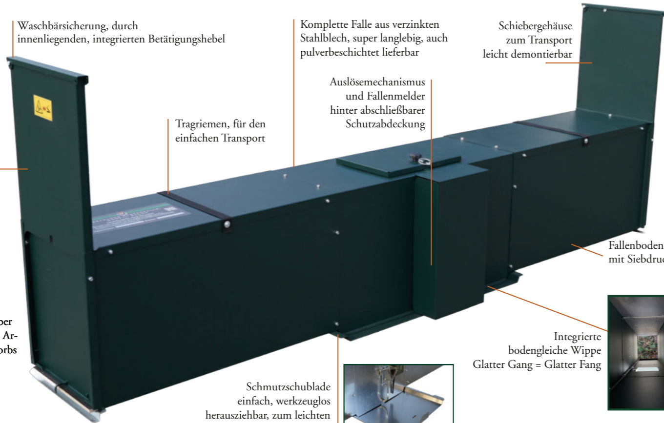
Deckel und Schutzgitter klappbar, auch bei Eis und Schnee einfach zu bedienen, Handschlitz zur Fangerkennung
